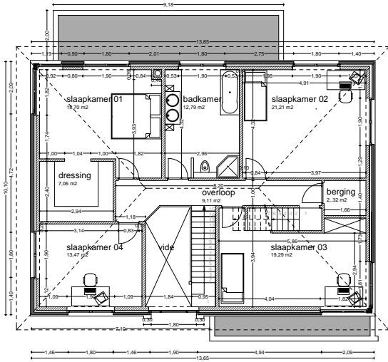
VERDIEPING
