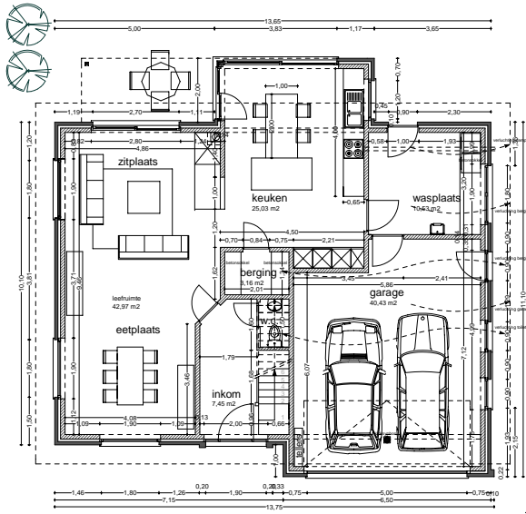
GELIJKVLOERS
