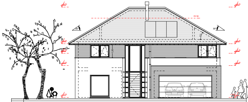
VOORGEVEL
