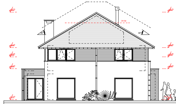
ZIJGEVEL LINKS
