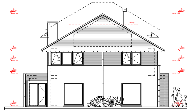
ZIJGEVEL LINKS
