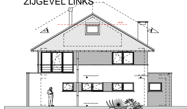
ZIJGEVEL RECHTS
