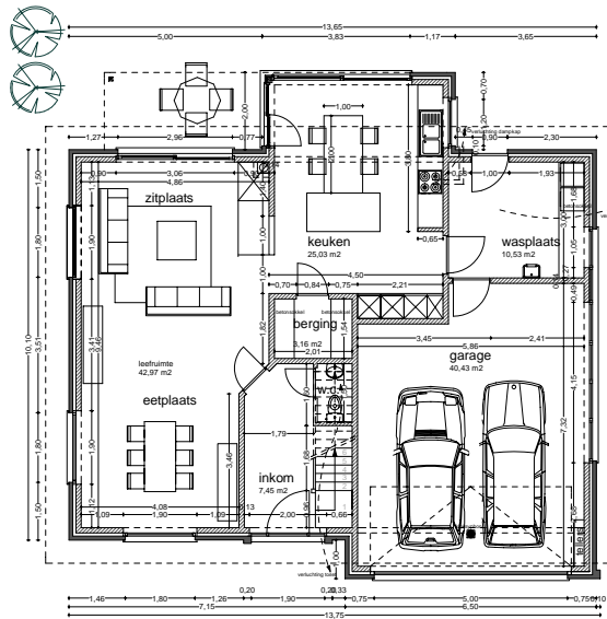
GELIJKVLOERS
