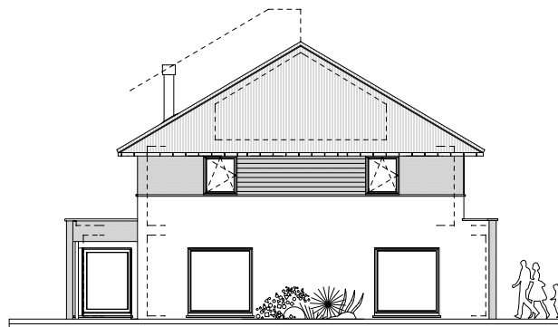
ZIJGEVEL LINKS
