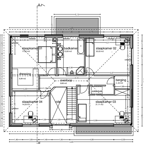
VERDIEPING
