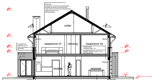
DOORSNEDEN A/A
