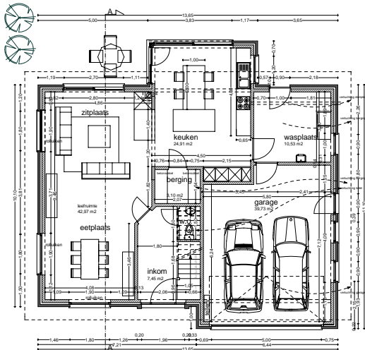
GELIJKVLOERS
