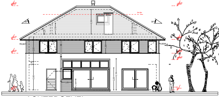
ACHTERGEVEL
