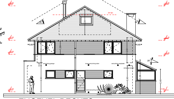
ZIJGEVEL RECHTS
