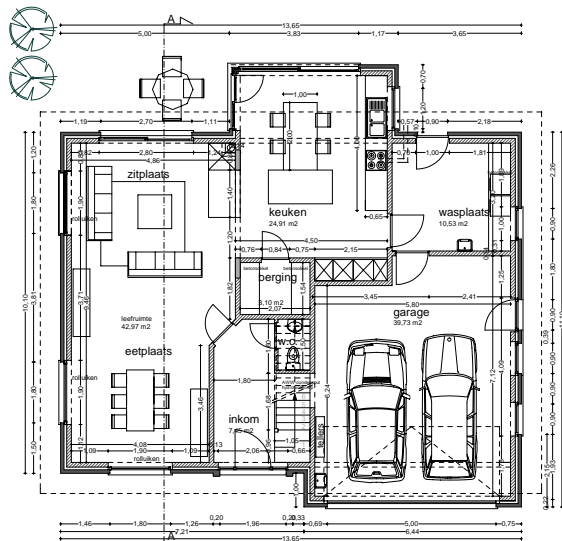
GELIJKVLOERS
