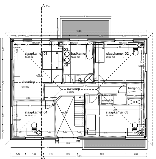
VERDIEPING
