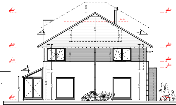
ZIJGEVEL LINKS
