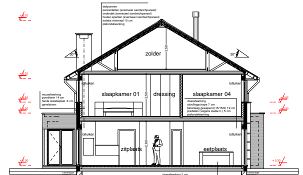
DOORSNEDEN A/A
