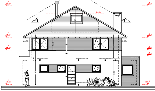
ZIJGEVEL RECHTS
