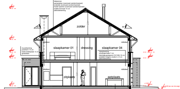
DOORSNEDEN A/A
