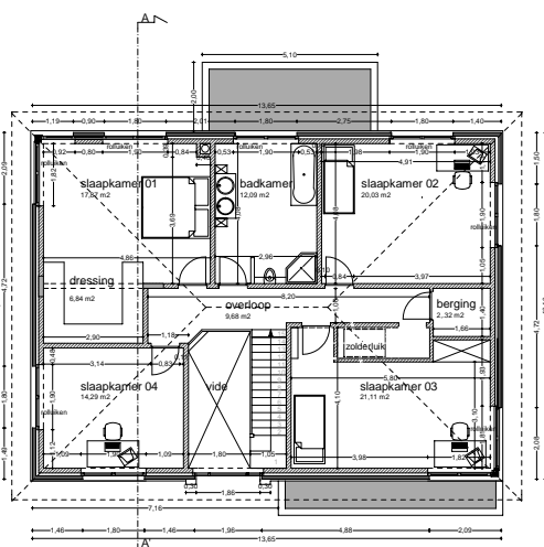
VERDIEPING
