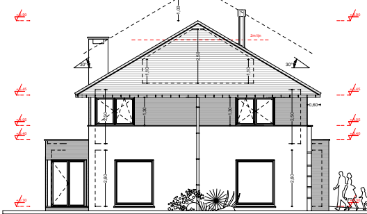
ZIJGEVEL LINKS
